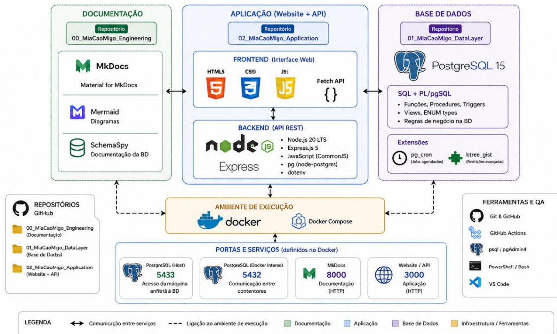
Figura 6 - Arquitetura técnica geral do sistema MiaCaoMiGo.
