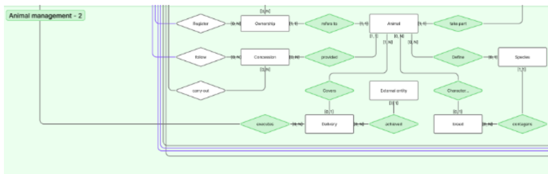
Figura 3 - Diagrama Entidade-Relação do módulo de Gestão do Ciclo de Vida Animal.
