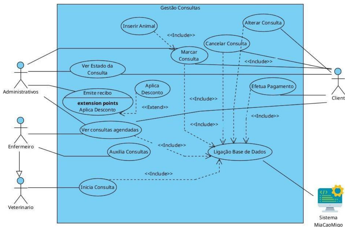
Figura 9 - Figura de CdU2 - Marcação de Consulta
