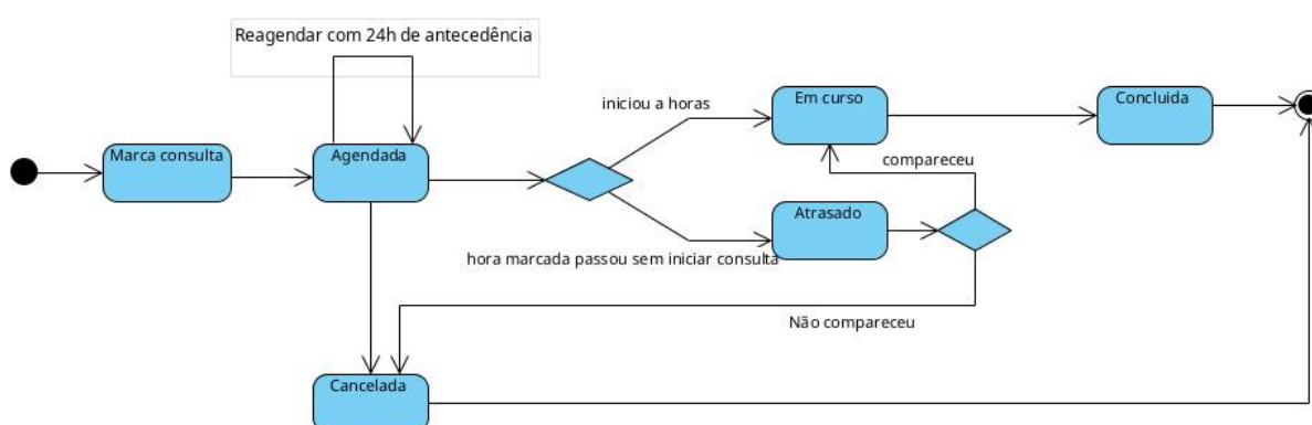
Figura 13 - Diagrama de estados de marcação de consulta
