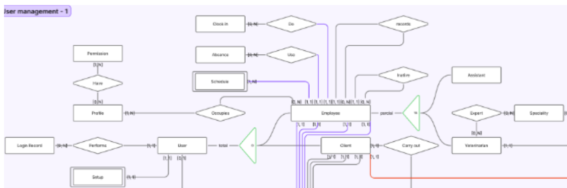
Figura 2 - Diagrama Entidade-Relação do módulo de Gestão Organizacional e Acessos.
